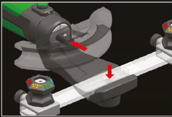
Bükme kalıbı ve üniversal traversin hızlı montajı
